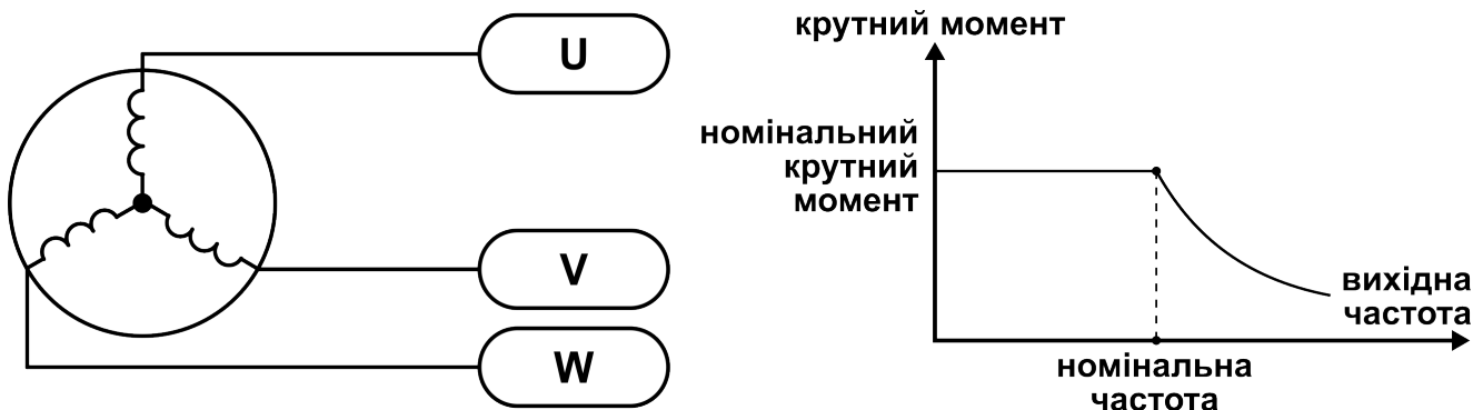
Рисунок 22. Трифазний асинхронний двигун.
