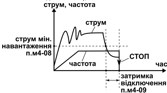
Рисунок 17. Принцип роботи захисту за мінімальним струмом двигуна.
