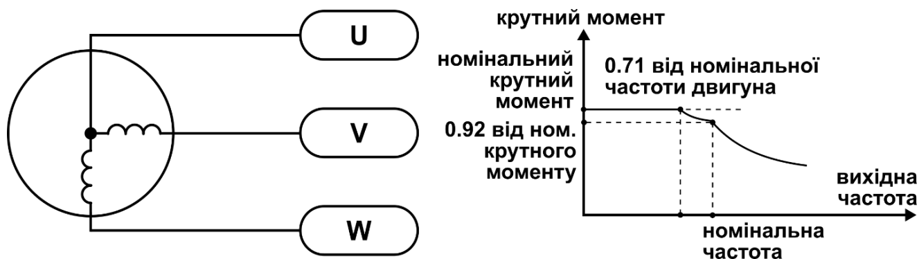
Рисунок 23. Однофазний двигун, підключений обома обмотками до ПЧ за трипровідною схемою.
