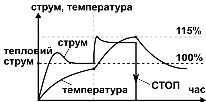
Рисунок 27. б) Принцип дії захисту від перегрівання двигуна.
